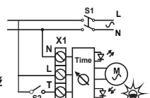
Elektrické schéma 2
