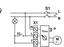
Elektrické schéma 4
